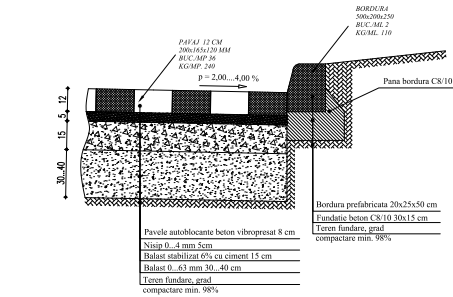
Secțiune transversală pavele auto trafic greu și intens
