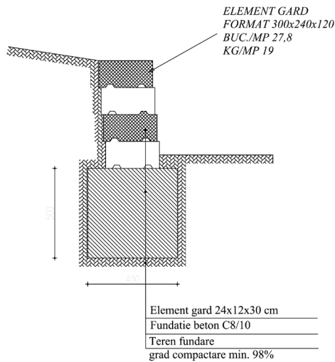
Secțiune transversală zid
