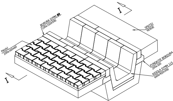
Vedere spațială montaj rigolă trapez
