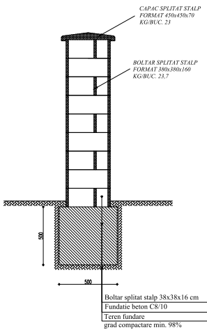
Secțiune transversală gard
