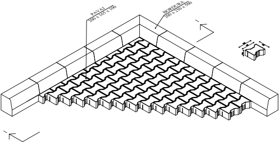
Vedere spațială pavele auto trafic greu
