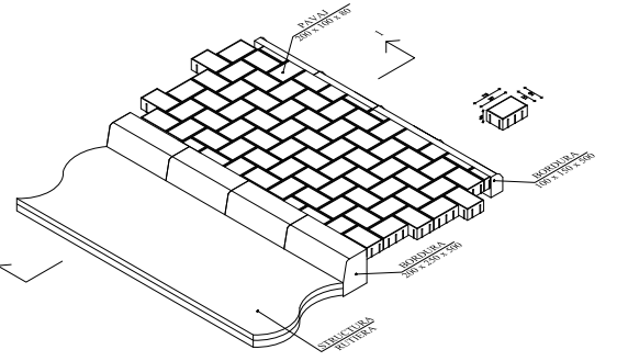
Vedere spațială pavele pietonale cu grosime de 8 cm
