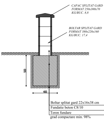
Secțiune transversală zid
