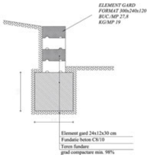
Secțiune transversală zid
