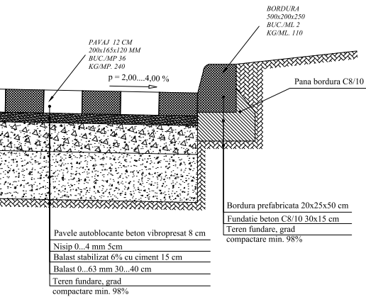
Secțiune transversală pavele auto trafic greu
