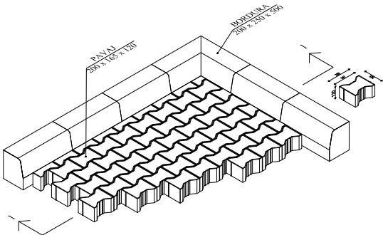
Vedere spațială pavele auto trafic greu și intens
