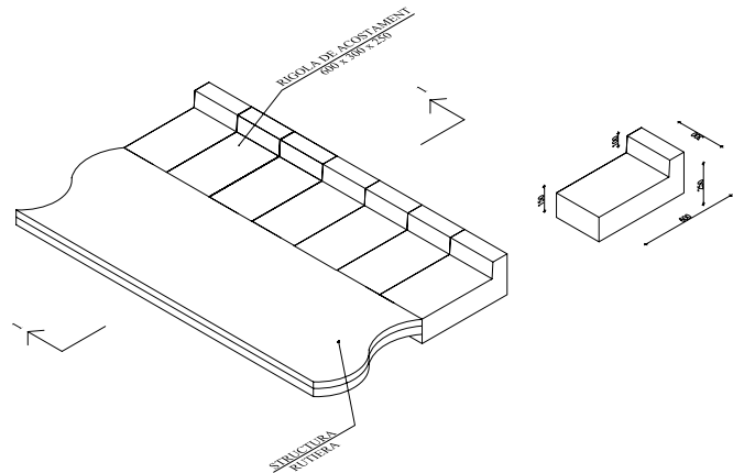
Vedere spațială rigole carosabile deschise
