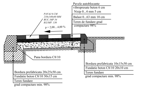
Secțiune transversală pavele pietonale cu grosime de 6 cm
