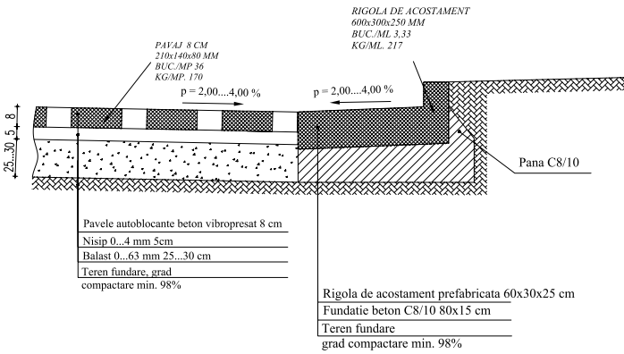
Vedere spațială rigole carosabile deschise
