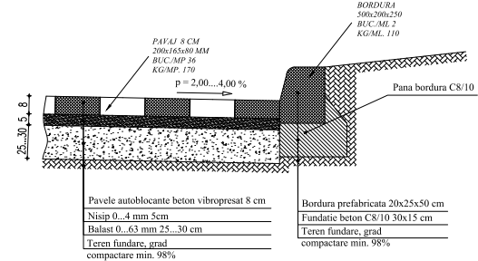
Secțiune transversală pavele auto trafic mediu
