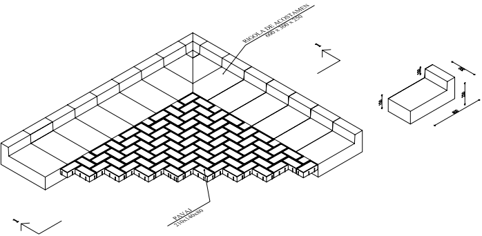
Secțiune transversală montaj pe piatră spartă
