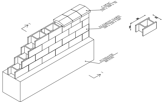
Vedere spațială zid
