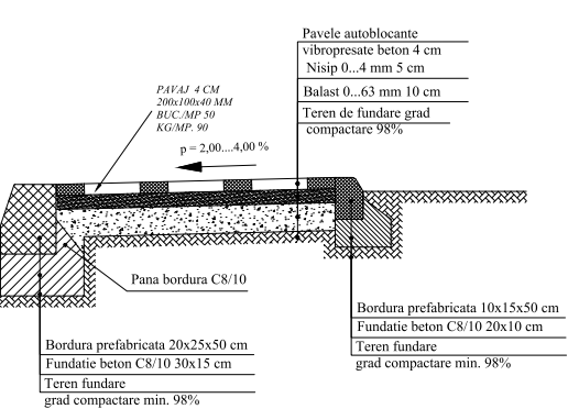
Secțiune transversală pavele pietonale cu grosime de 4 cm
