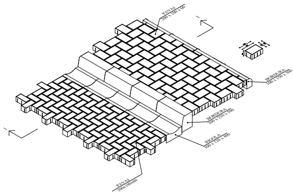
Secțiune transversală rigole carosabile deschise
