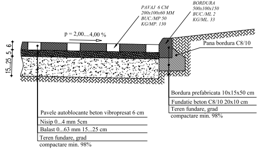
Vedere spațială pavele auto trafic mediu
