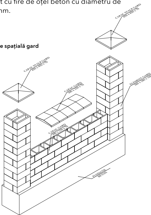
Vedere spațială gard
