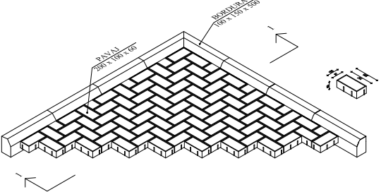
Secțiune transversală pavele auto trafic ușor
