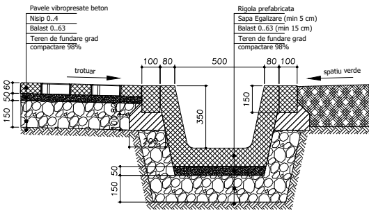
Secțiune transversală montaj rigolă trapez
