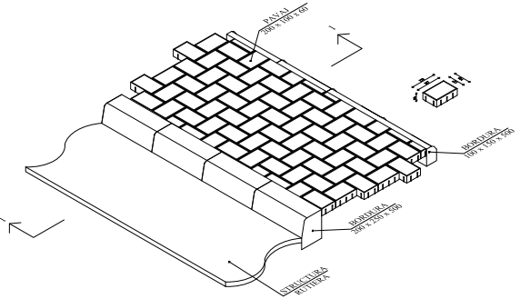
Vedere spațială pavele pietonale cu grosime de 6 cm
